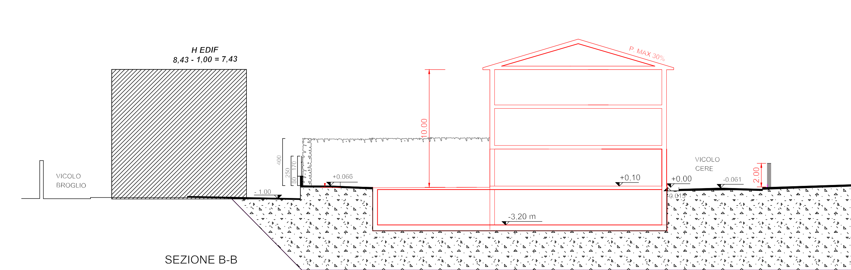
SEZIONE B-B
